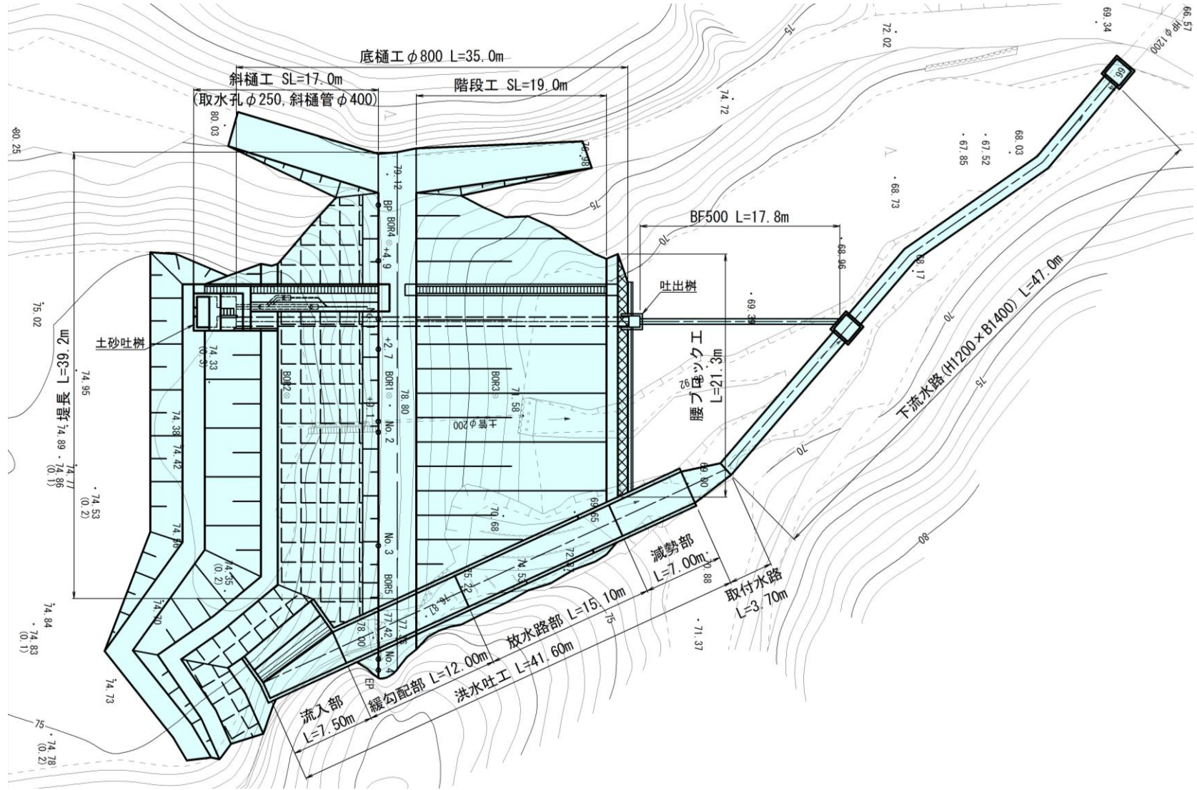
計画平面図
