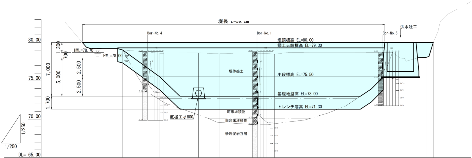
縦断図
