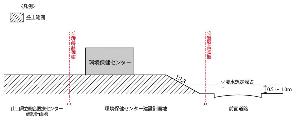
図 3.2.1 造成イメージ図
