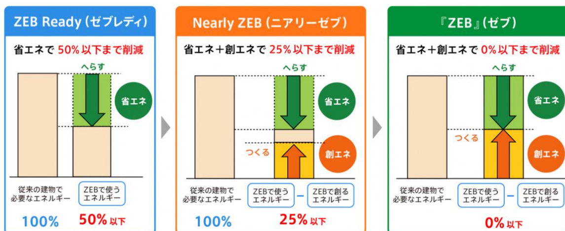
図 3.5.1 ZEB 化のイメージ（出典：ZEB PORTAL（ゼブ・ポータル）のウェブサイト（環境省））
