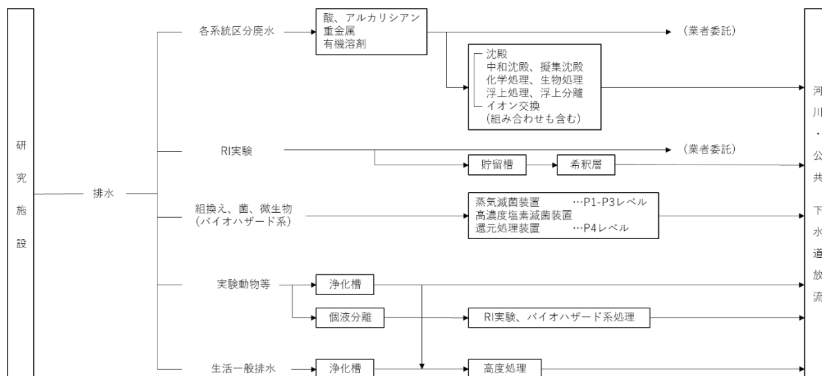
図 2.4.1 排水処理フローのイメージ
