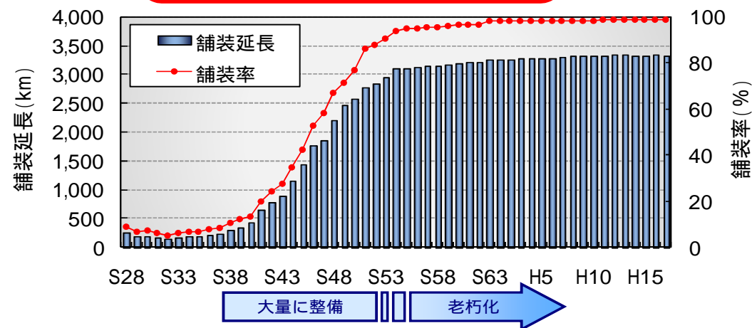
舗装延長と舗装率の推移
