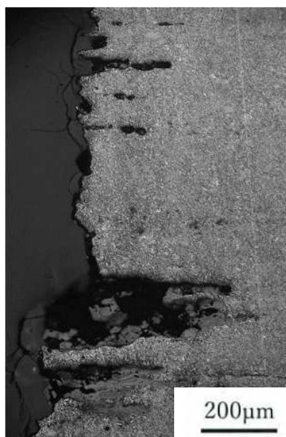
(e)中心部 100 倍
