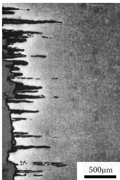
(d)中心部 50 倍
