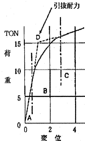
図4-1 ロックボルト引抜試験
