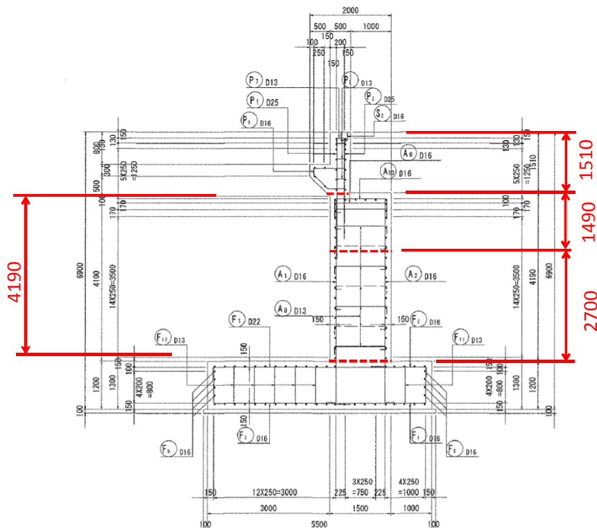
配筋図
