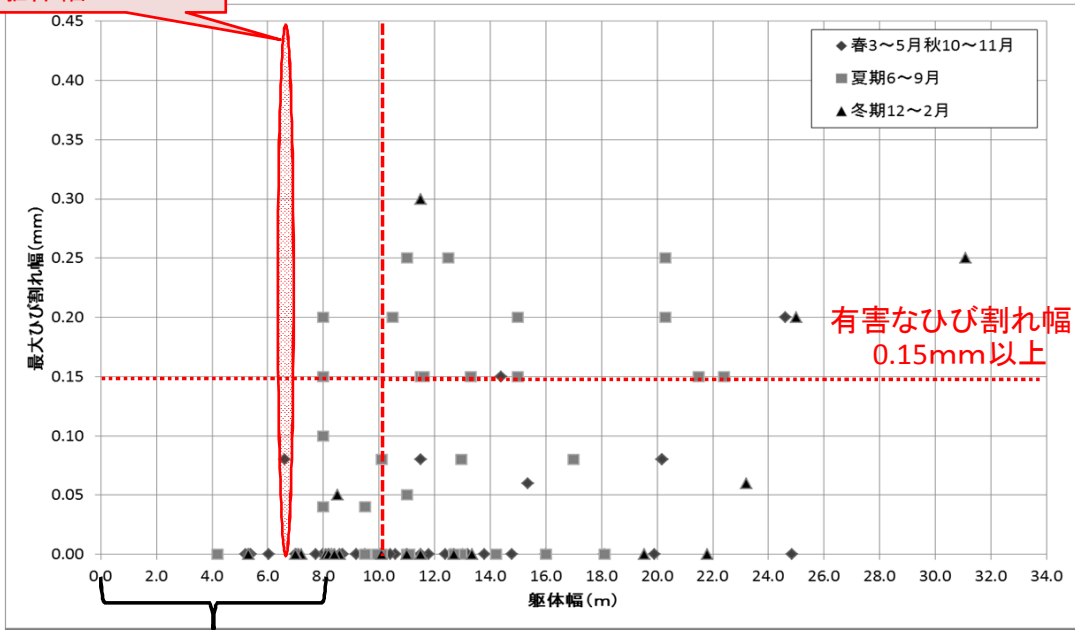
躯体幅と最大ひび割れ幅の関係
