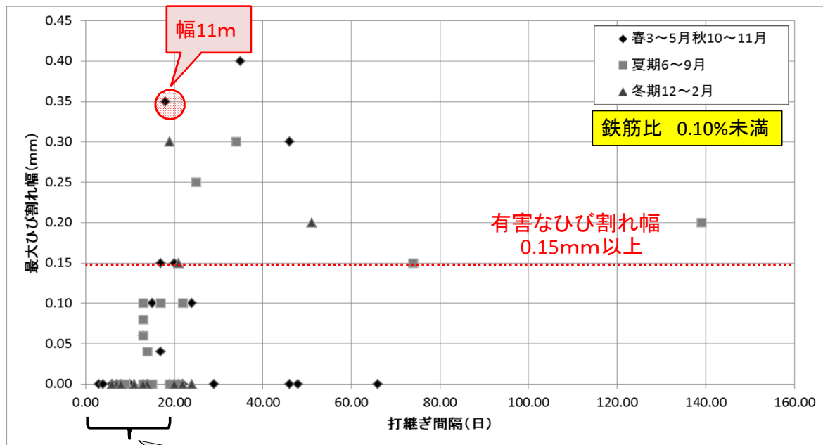
打継ぎ間隔と最大ひび割れ幅の関係(類似の鉄筋比)
