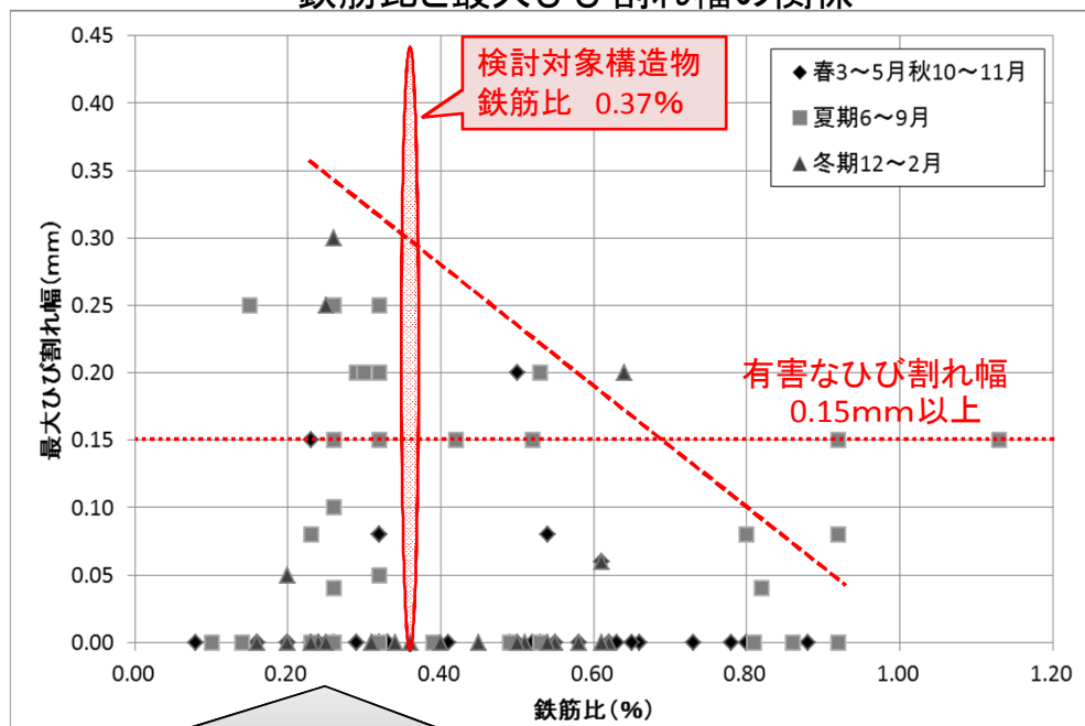
鉄筋比と最大ひび割れ幅の関係
