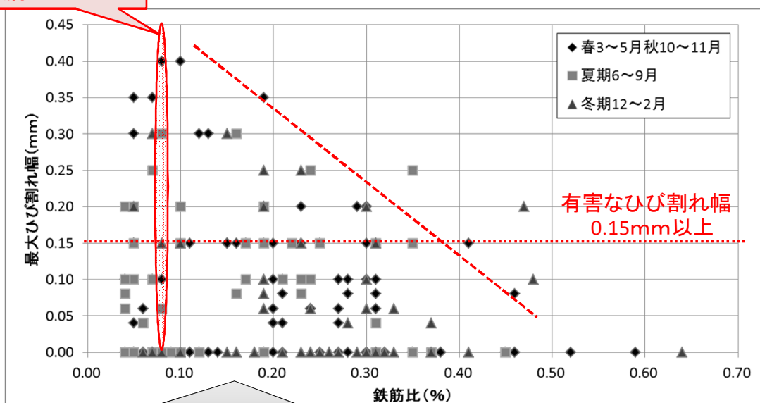
鉄筋比と最大ひび割れ幅の関係
