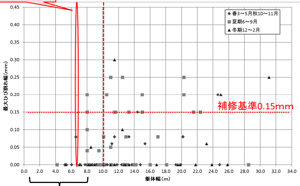
躯体幅と最大ひび割れ幅の関係
