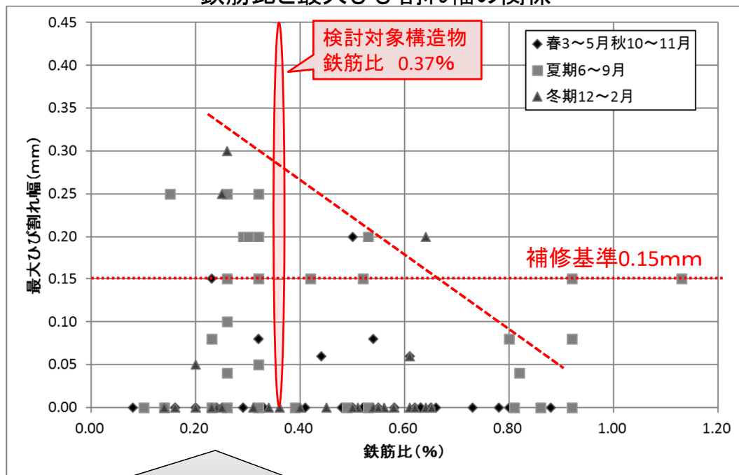
鉄筋比と最大ひび割れ幅の関係
