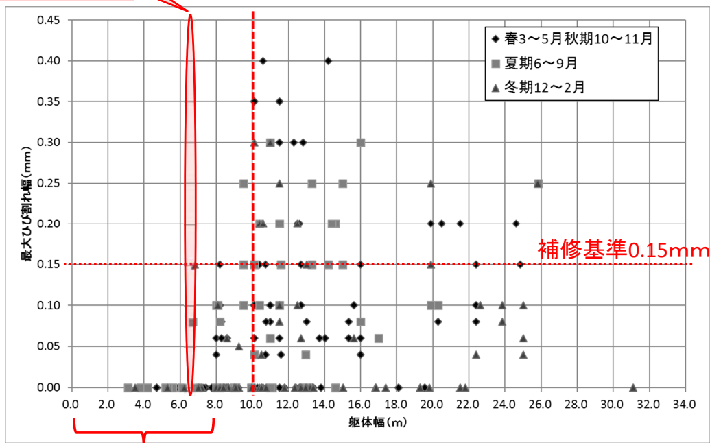
躯体幅と最大ひび割れ幅の関係
