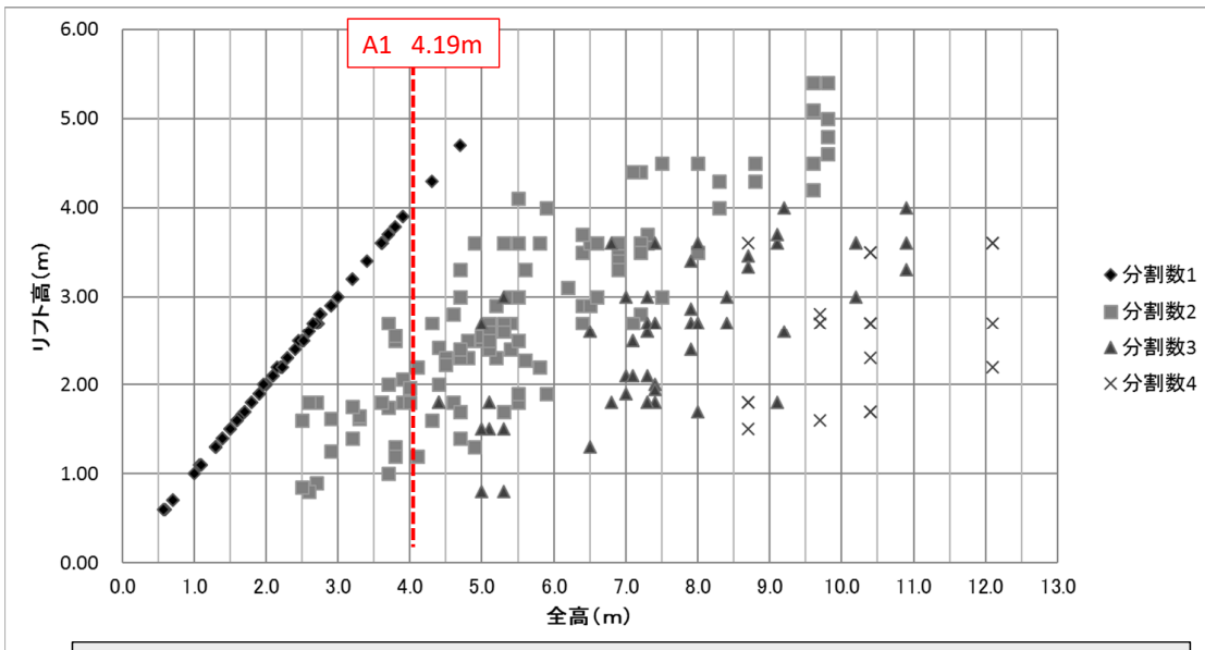
たて壁全高とリフト高(分割数)の関係
