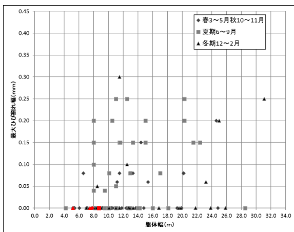
図-3 橋台胸壁における 躯体幅と最大ひび割れ幅の関係
