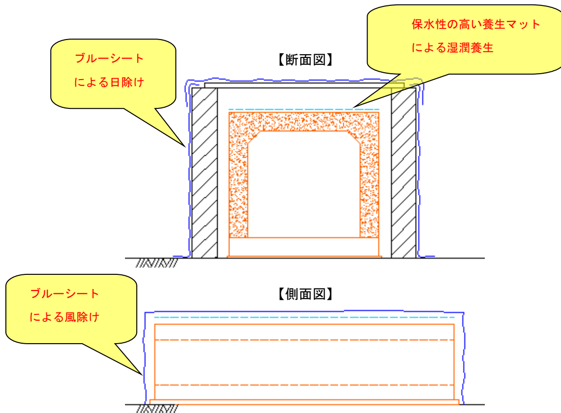
図 3.3.17 保護養生概要図
