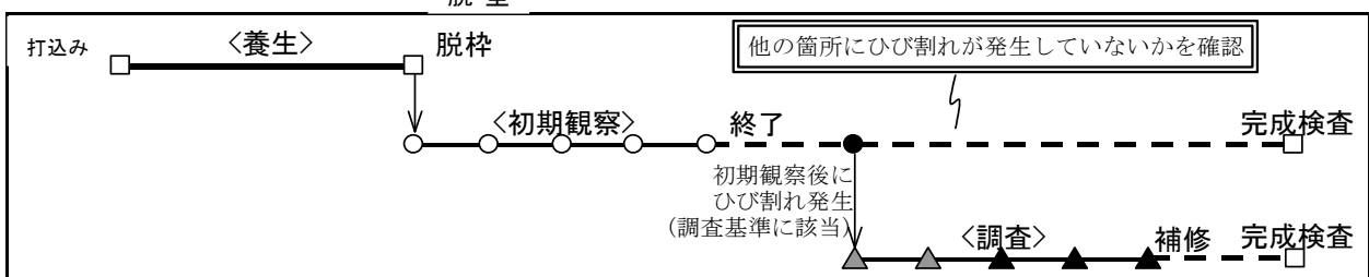
⑤初期観察後に発生したひび割れが調査基準に該当し、調査終了までに補修基準にも該当する場合
