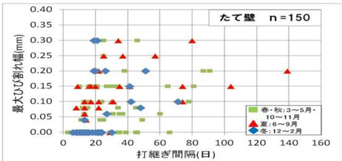
図 3.3.2 打継ぎ間隔と最大ひび割れ幅（橋台たて壁）
