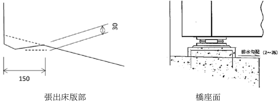
図. 3. 4. 1 橋梁の水切り・排水構造の例
