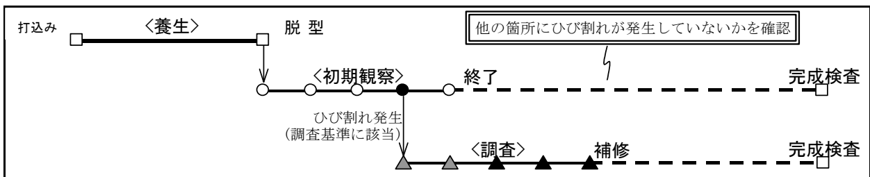
④観察中に発生したひび割れが調査基準に該当し、調査終了までに補修基準にも該当する場合
