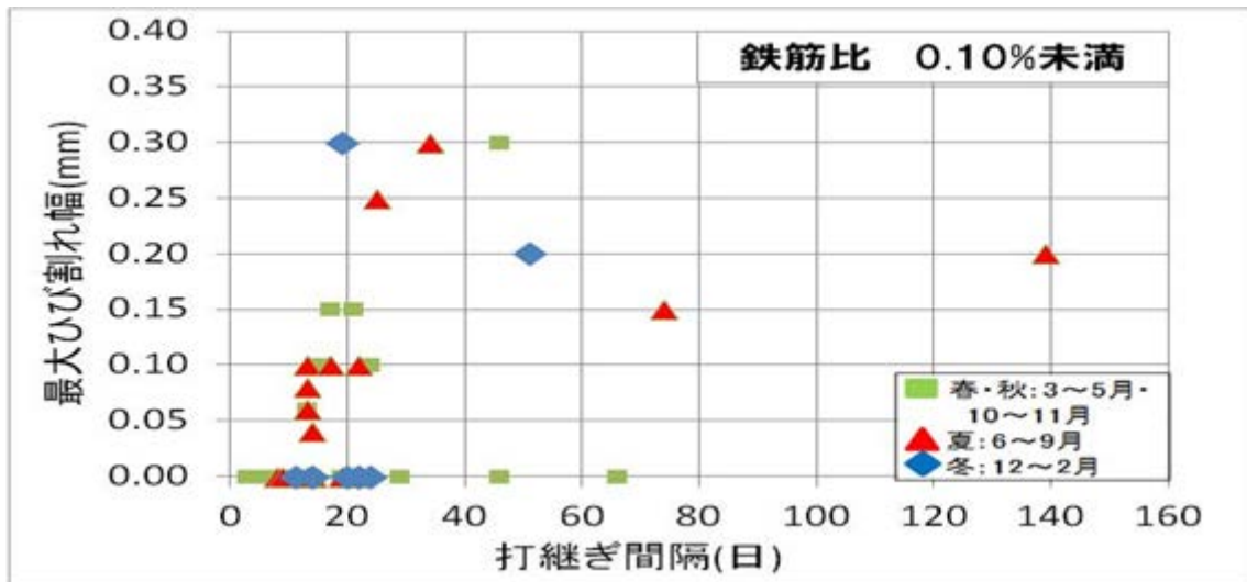
図 3.3.4 打継ぎ間隔と最大ひび割れ幅（橋台たて壁 鉄筋比 0.10%未満）
