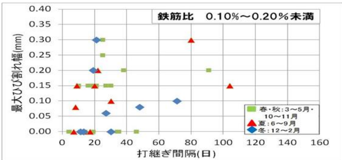
図 3.3.5 打継ぎ間隔と最大ひび割れ幅（橋台たて壁 鉄筋比 0.10%~0.20%未満）
