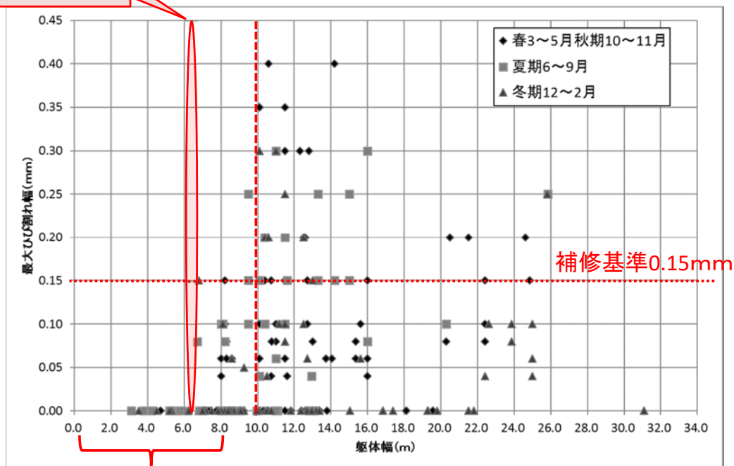
躯体幅と最大ひび割れ幅の関係
