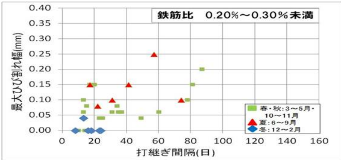
図 3.3.6 打継ぎ間隔と最大ひび割れ幅（橋台たて壁 鉄筋比 0.20%～0.30%未満）
