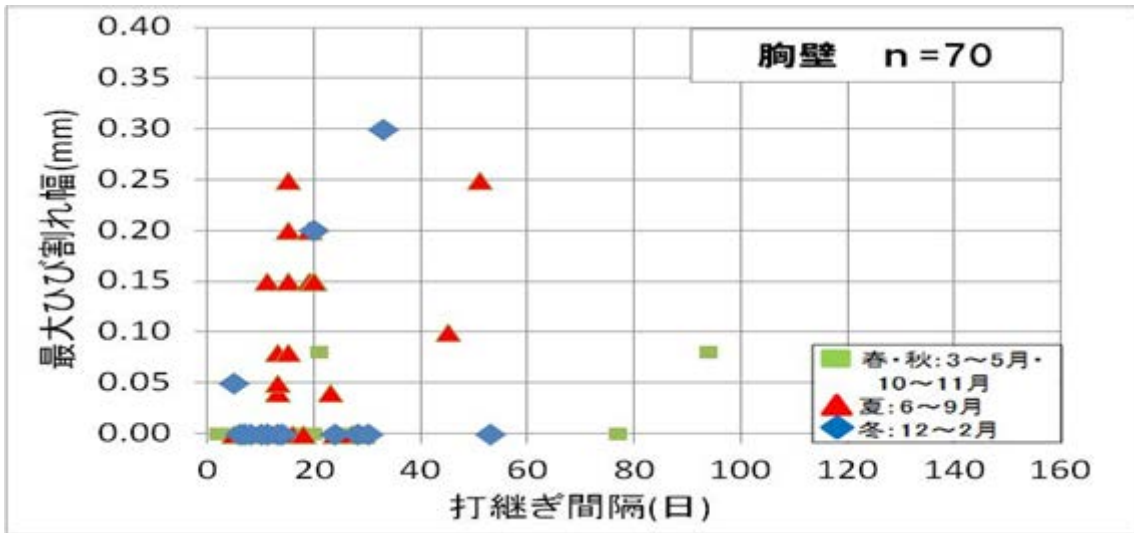
図 3.3.3 打継ぎ間隔と最大ひび割れ幅（橋台胸壁）
