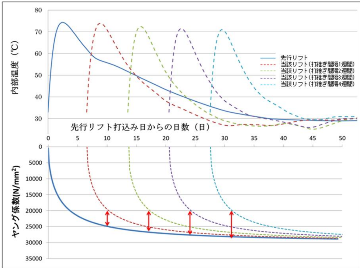
図 3.3.9 コンクリートの打継ぎ後経過日数と内部温度、ヤング係数の変化
