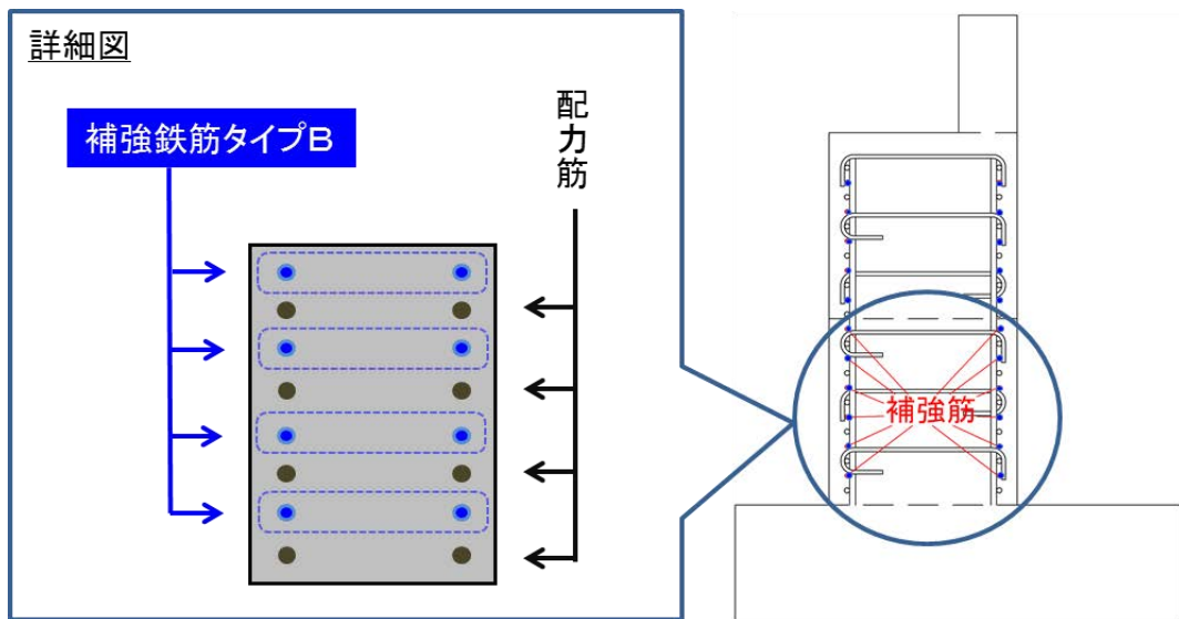
図 3.3.13 ひび割れ発生方向と抵抗鉄筋概要図 (補強鉄筋タイプB)
