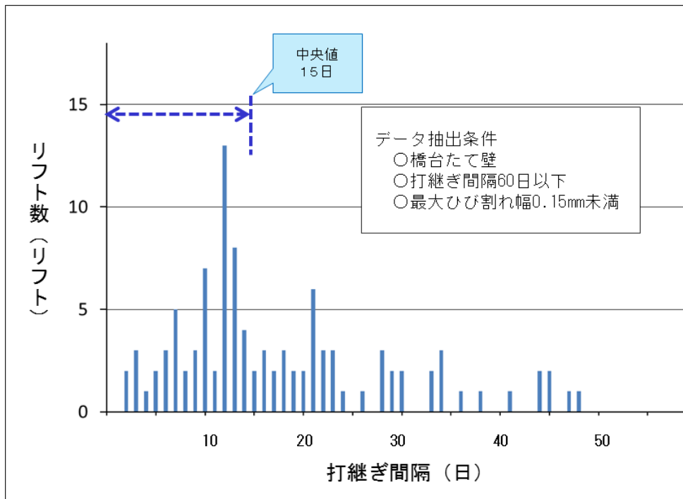
図 3.3.10 打継ぎ間隔と最大ひび割れ幅が0.15mm未満のリフト数
