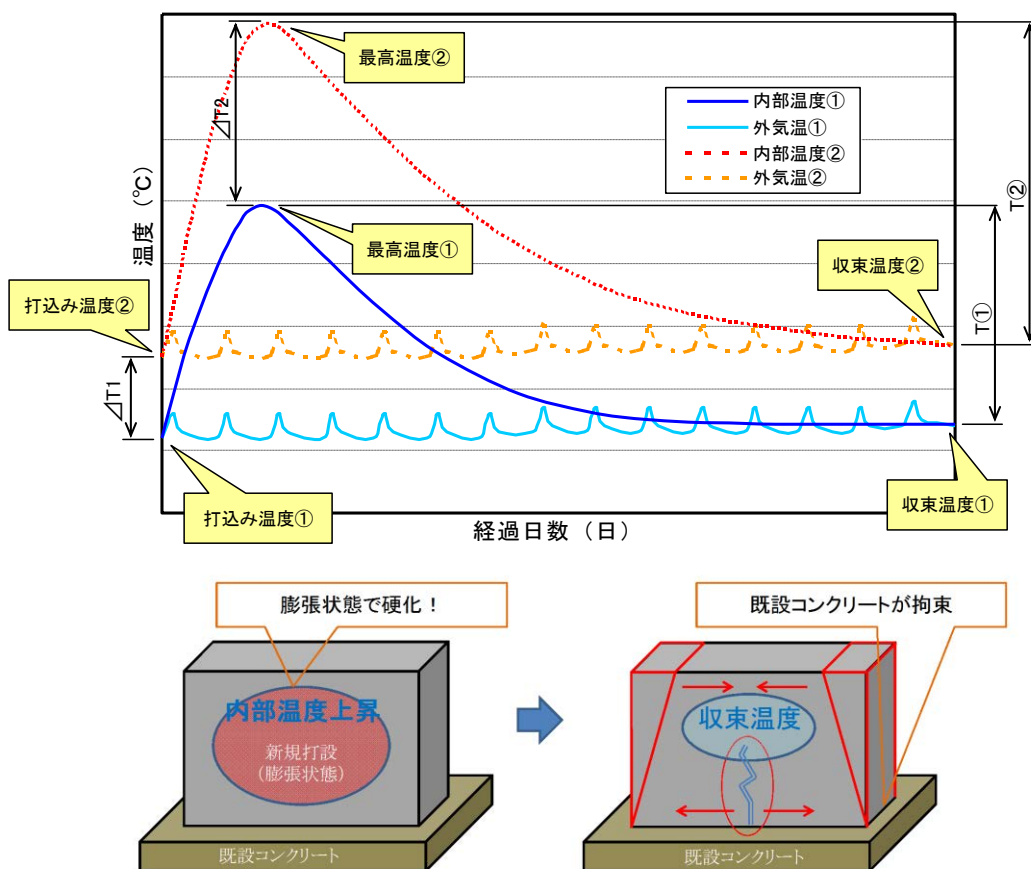
図 3.3.1 コンクリート内部温度の経時変化
