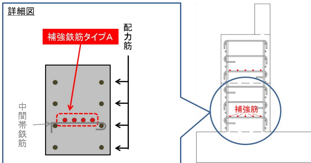
図 3.3.12 ひび割れ発生方向と抵抗鉄筋概要図 (補強鉄筋タイプ A)
