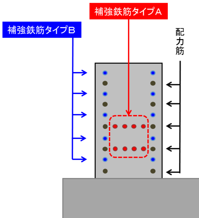
図 3.3.14 補強鉄筋タイプ A+B
