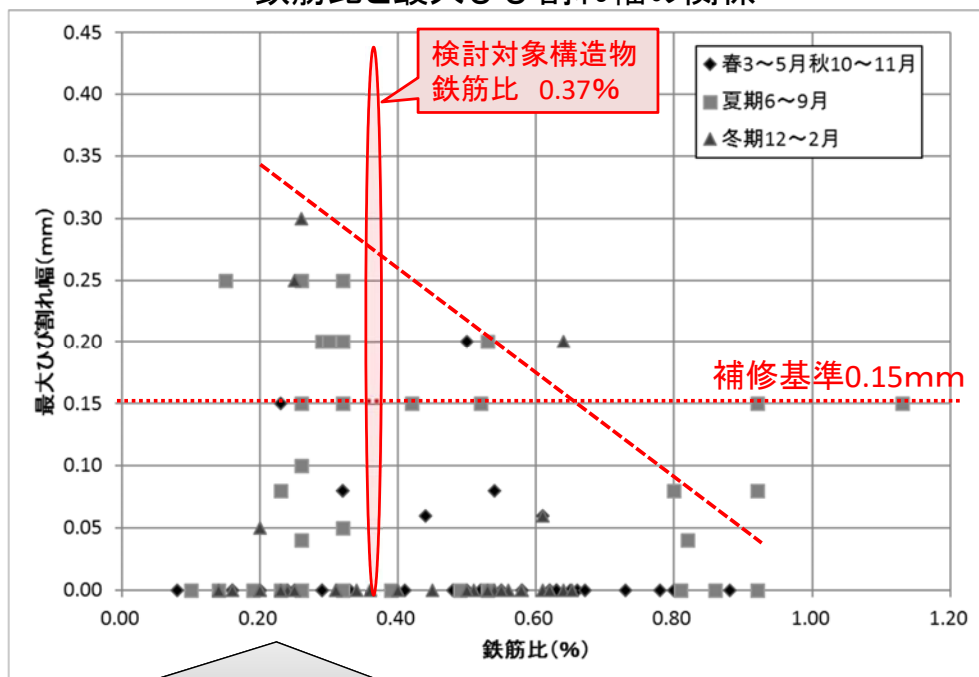
鉄筋比と最大ひび割れ幅の関係
