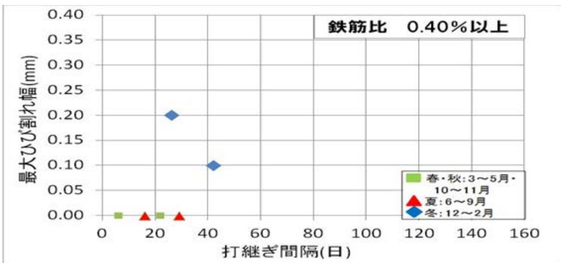
図 3.3.8 打継ぎ間隔と最大ひび割れ幅（橋台たて壁 鉄筋比 0.40%以上）
