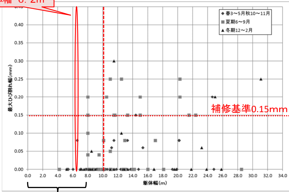
躯体幅と最大ひび割れ幅の関係
