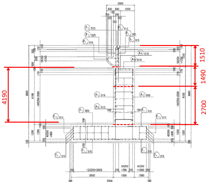
配筋図
