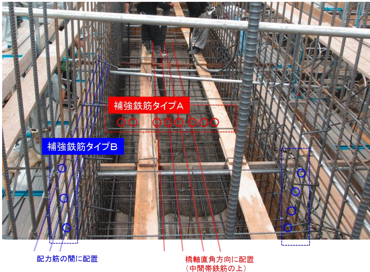
図 3.3.11 補強鉄筋配置状況図
