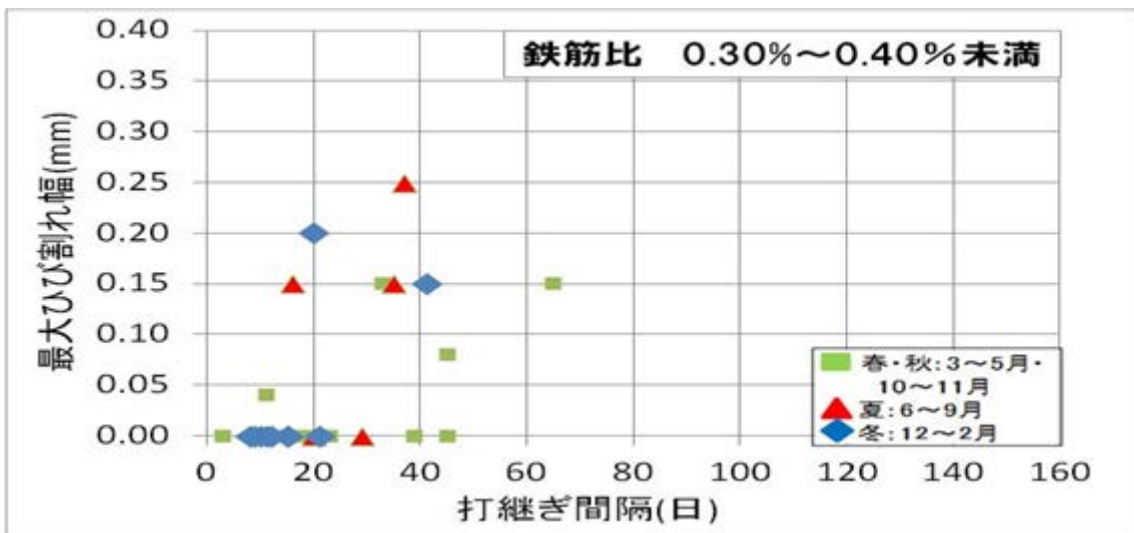
図 3.3.7 打継ぎ間隔と最大ひび割れ幅（橋台たて壁 鉄筋比 0.30%～0.40%未満）
