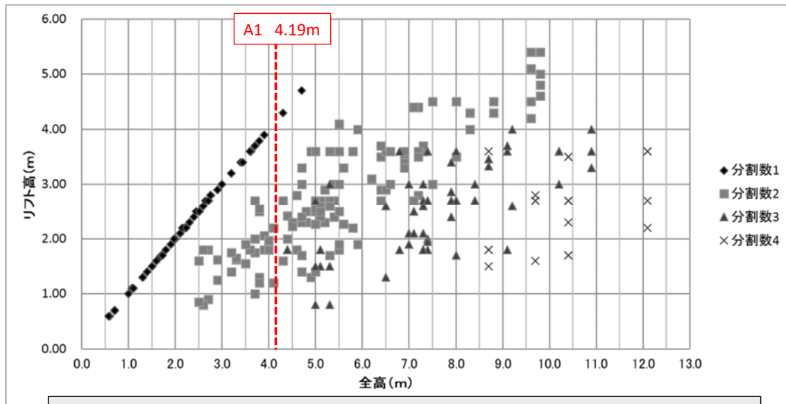
たて壁全高とリフト高(分割数)の関係
