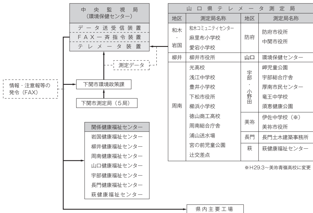
図4-10 山口県大気汚染監視測定網
