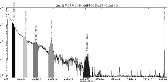
図 3 2015 年 7 月 14 日 6:30 30.6 nGy/h
