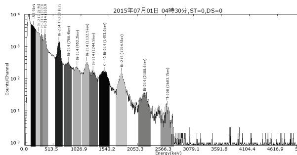
図 2 2015 年 7 月 1 日 4:30 98.0 nGy/h
