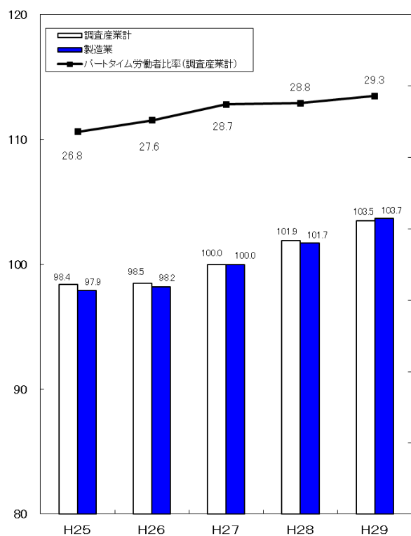
図7 (5人以上)
