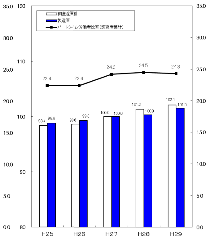
図8 (30人以上)
