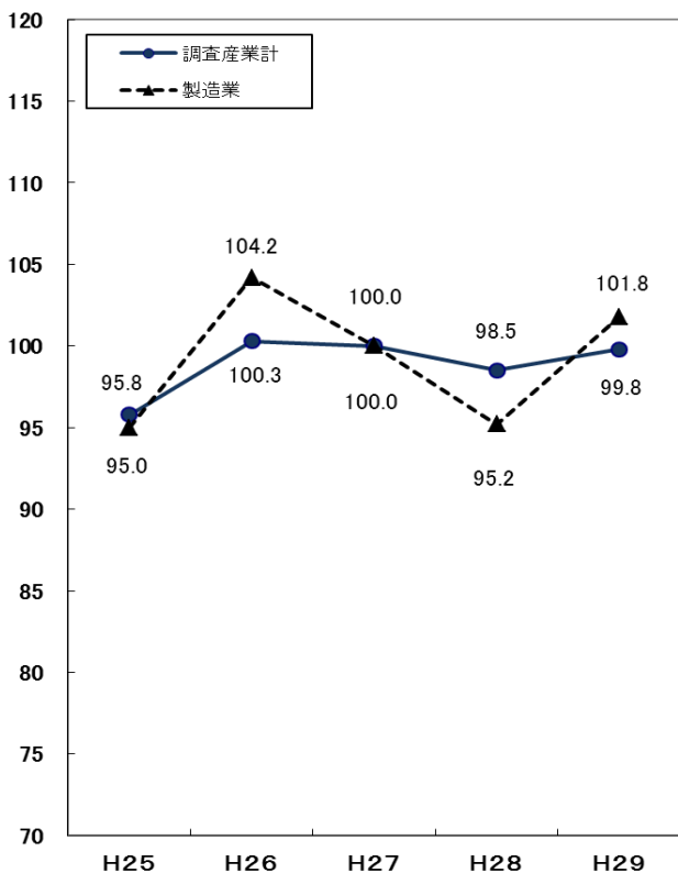
図5 (5人以上)
