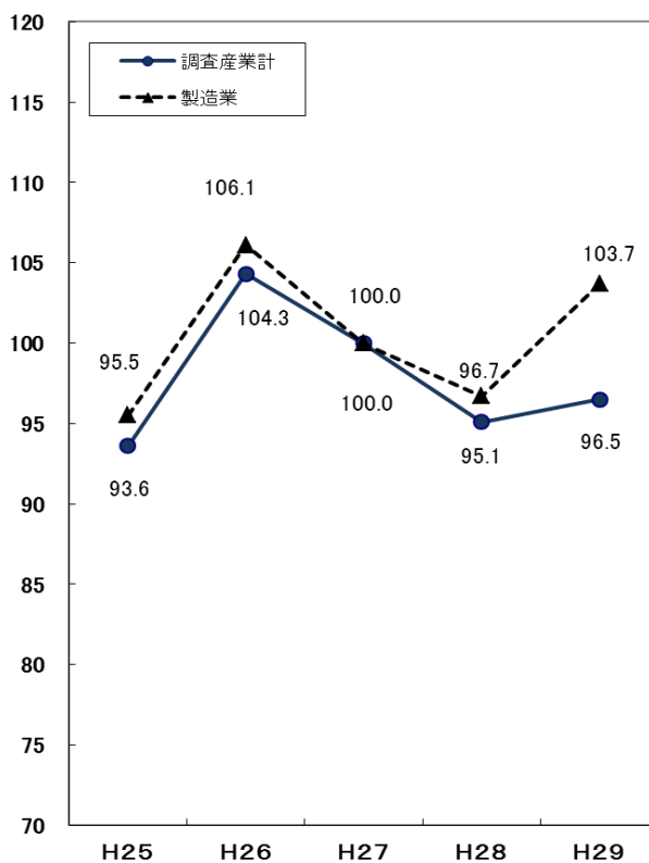
図6 (30人以上)
