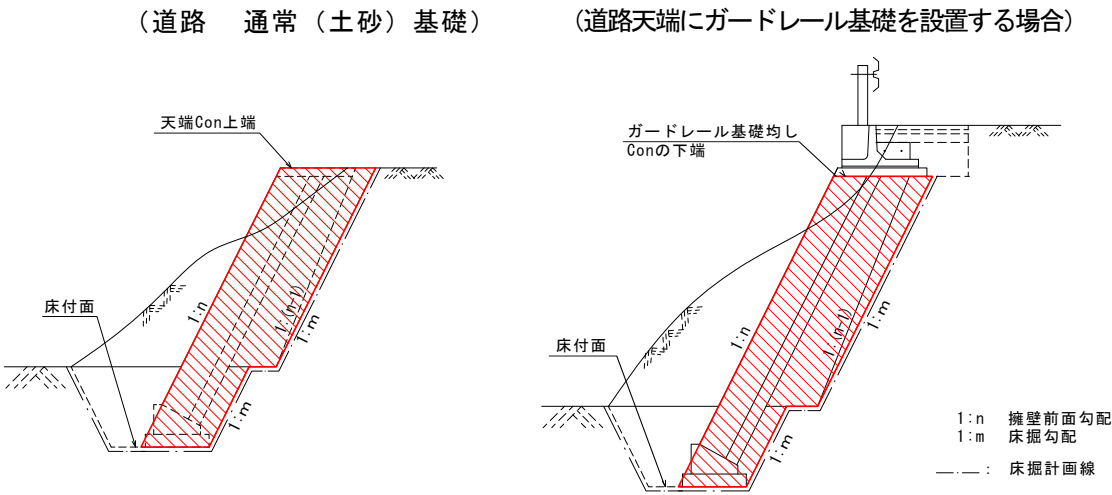
小口止工構造図 (参考)
