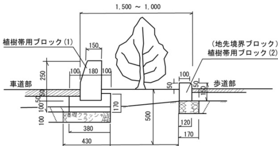
植樹帯用ブロック設置工 植樹帯標準断面図
