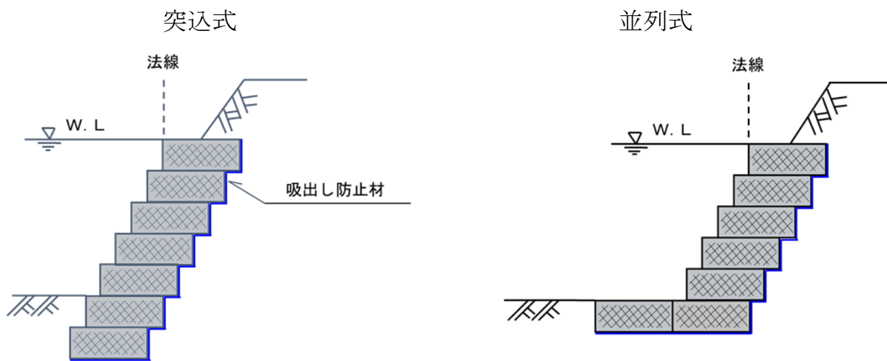
標準図
