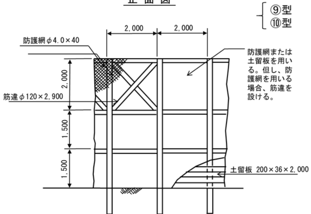
正面図
