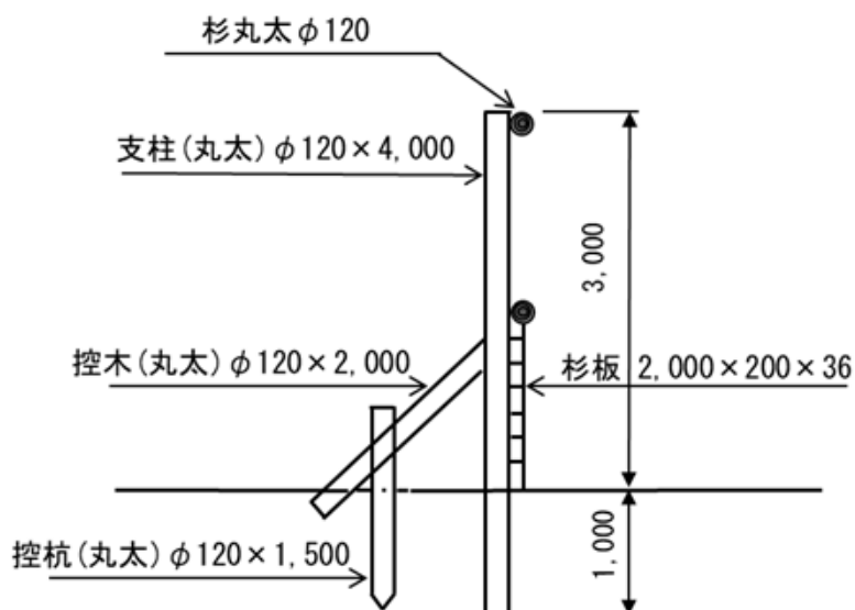
側面図
