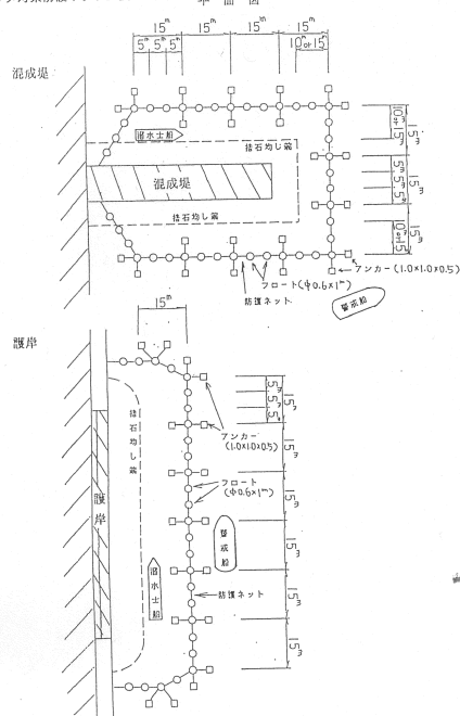
サメ対策防護ネット工法
