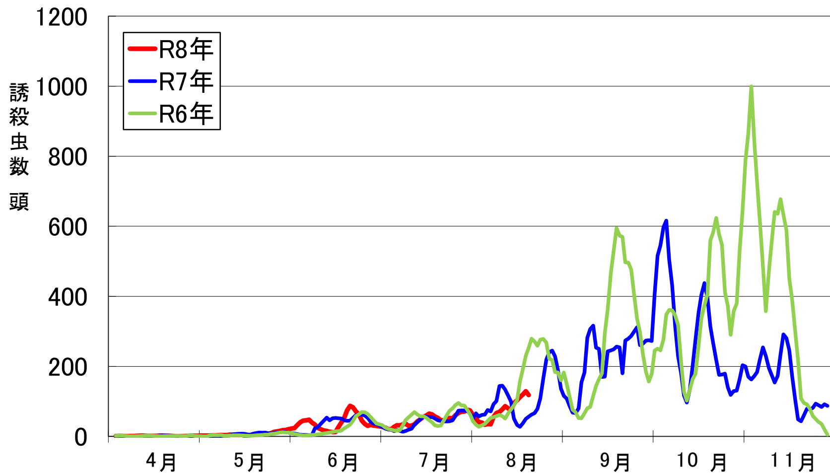
ハスモンヨトウフェロモントラップ誘殺数(移動平均)防府市牟礼
