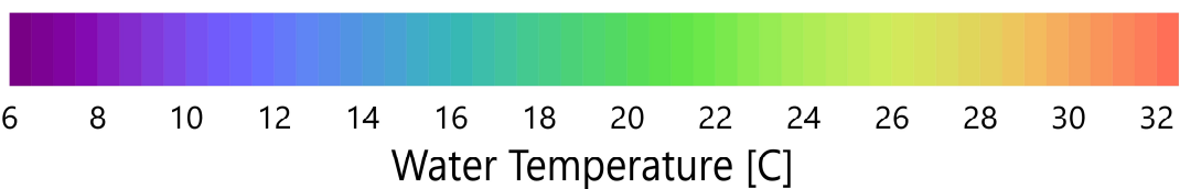
図. 水温の水平分布図 (2026年5月7・11・12日観測)
