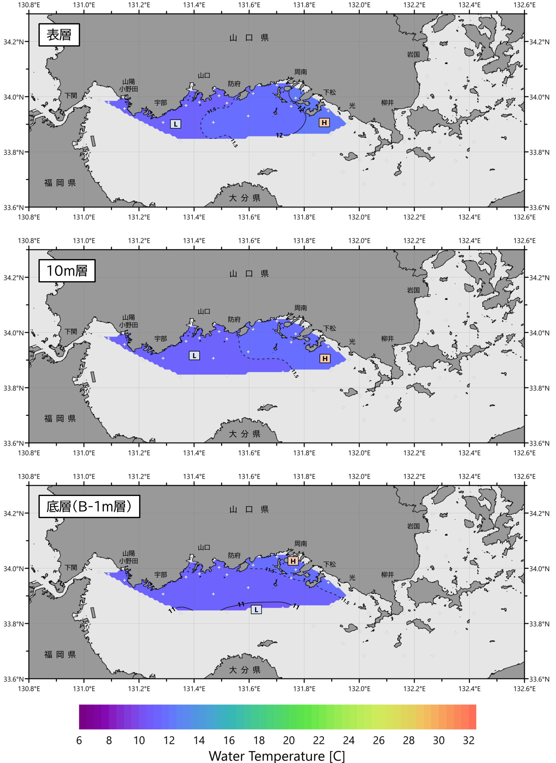
図. 水温の水平分布図 (2026年3月5日観測)
