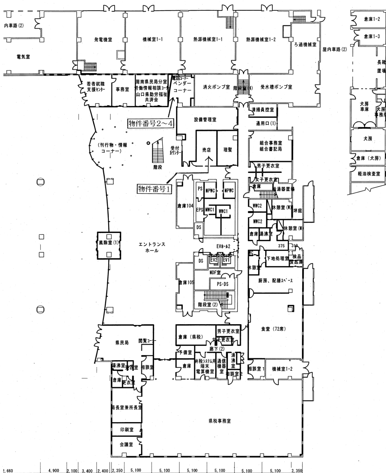
周南総合庁舎 1階平面図
