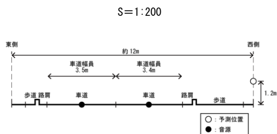
図 11. 2. 3-3 (3) 予測断面図 (③下関市彦島迫町 2 丁目 : 県道南風泊港線)
