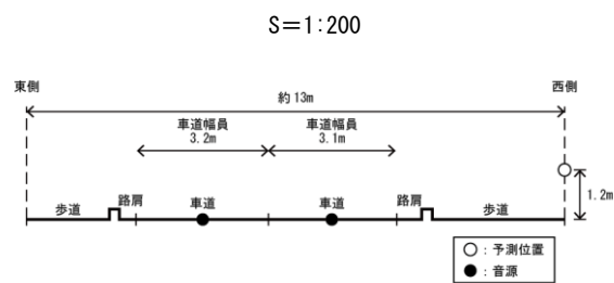
図 11. 2. 3-3 (2) 予測断面図 (②下関市彦島迫町 5 丁目 : 市道宮の前線)
