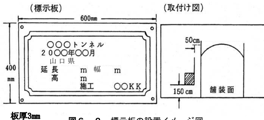
図6-2 標示板の設置イメージ図
