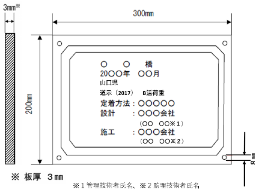
図 2-2 銘板の寸法及び記載事項
