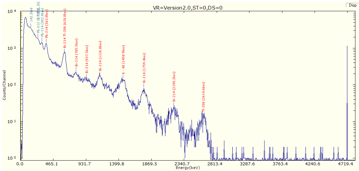
図1 平成26年1月8日 19:10 74.7nGy/h (最高値時のスペクトル)
