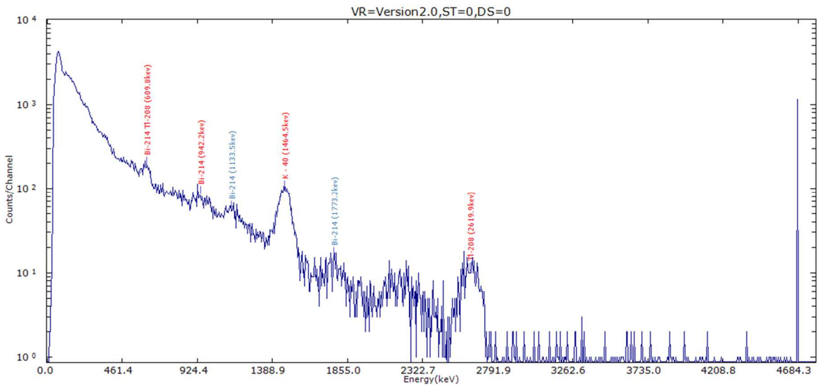
図2 平成26年3月9日 12:10 35.7nGy/h (最小値時のスペクトル)
