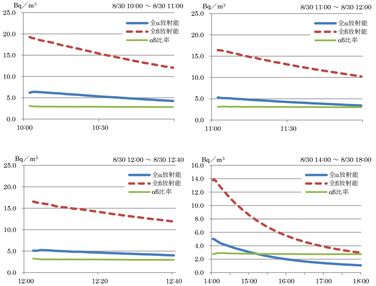
図3 全 \alpha ・ \beta 放射能の減衰(8月30日)
