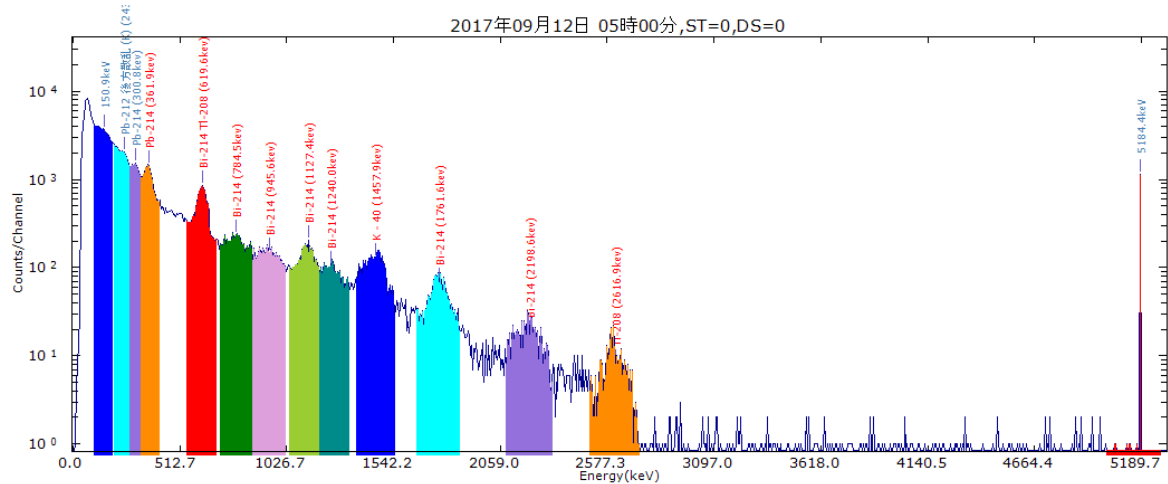
図1 平成29年9月12日 5:00 66.0nGy/h (最高値時のスペクトル)
