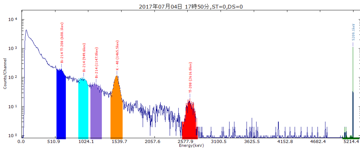
図2 平成29年7月4日 17:50 30.4nGy/h (最小値時のスペクトル)
