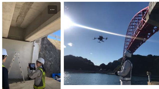
<橋梁点検の状況>
