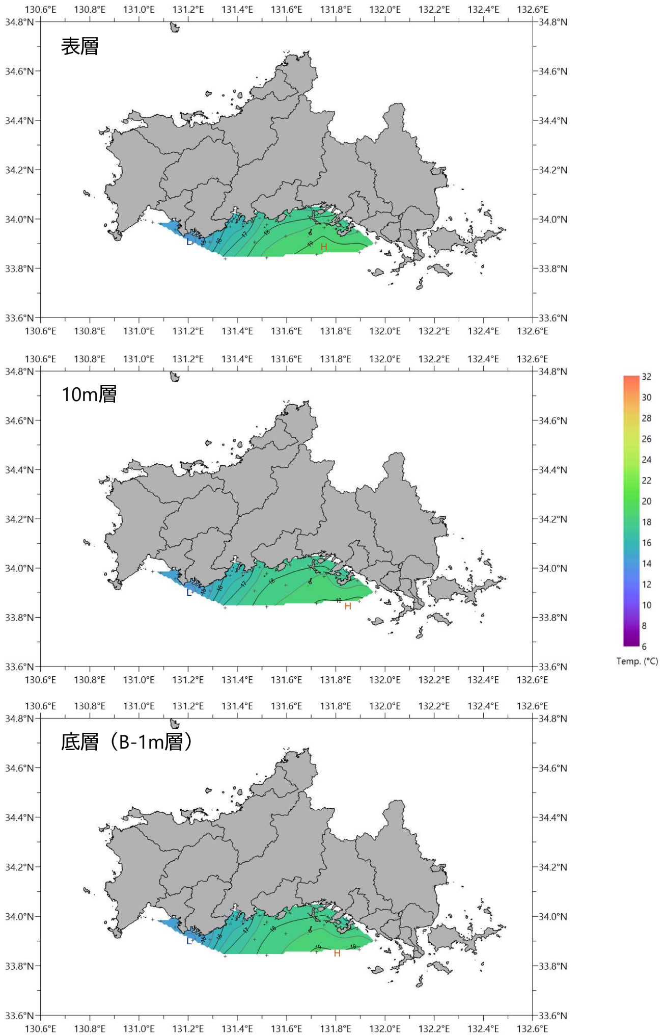
図. 水温の水平分布図(2024年12月2日観測)
