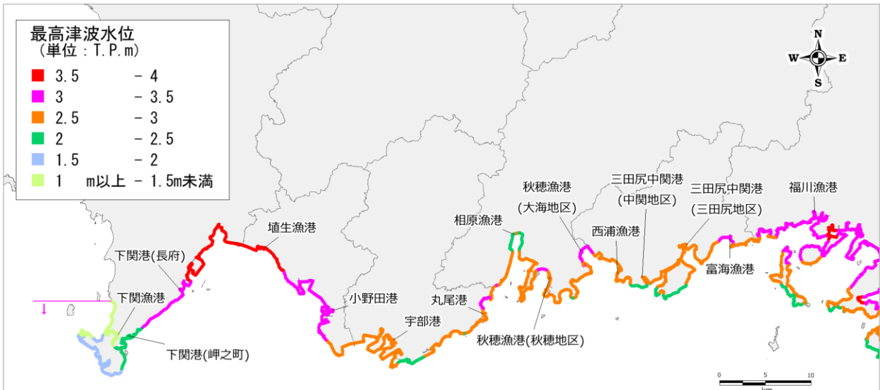
図 3 最高津波水位分布（西部）
