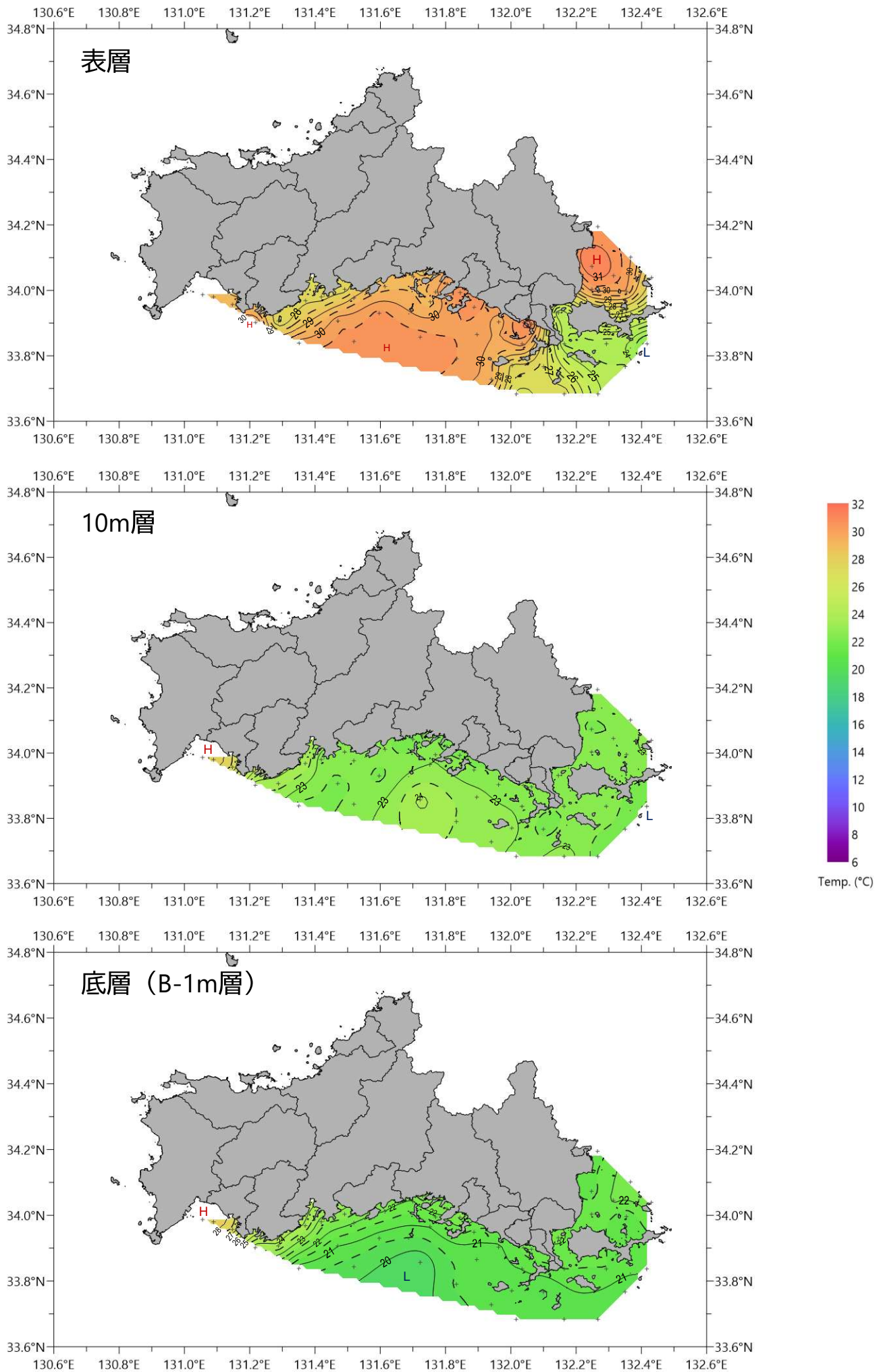
図. 水温の水平分布図(2024年8月5-6日観測)
