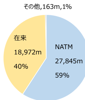
図 2-4 工法別の内訳・トンネル延長(令和 5 年 3 月現在)
