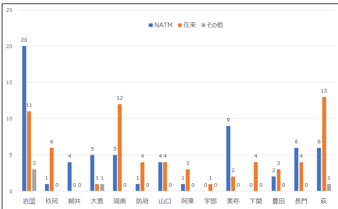
図 2-6 事務所別のトンネル数と整備工法の内訳（令和 5 年 3 月現在）
