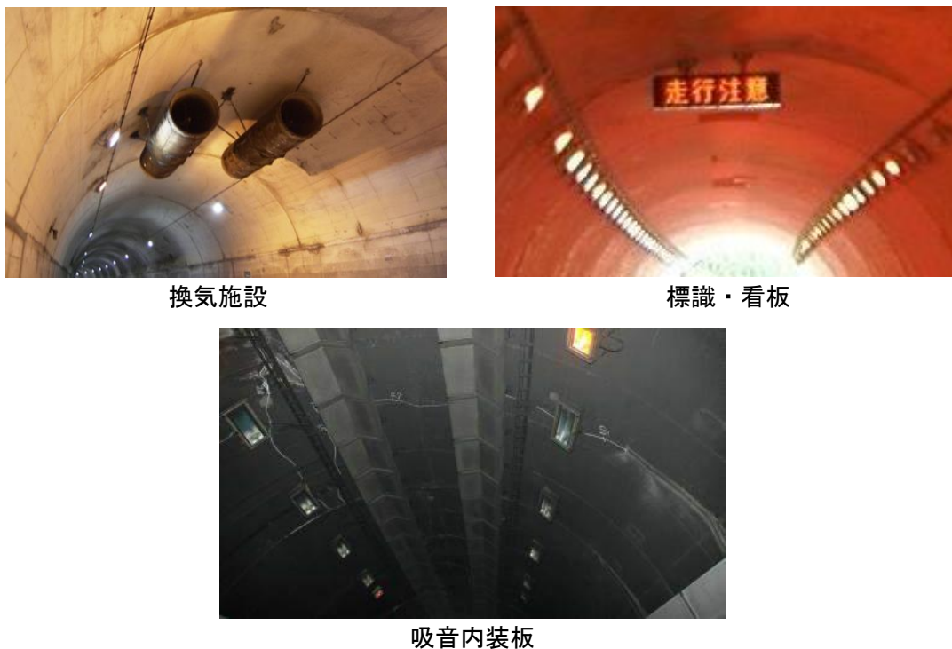
図 2-8 トンネル附属物の事例
