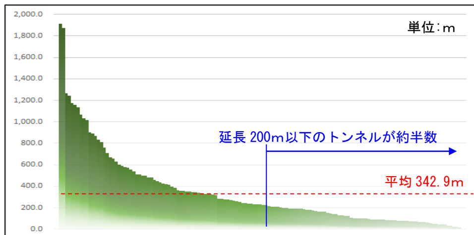
図 2-2 トンネル延長の一覧 (令和 5 年 3 月現在)
