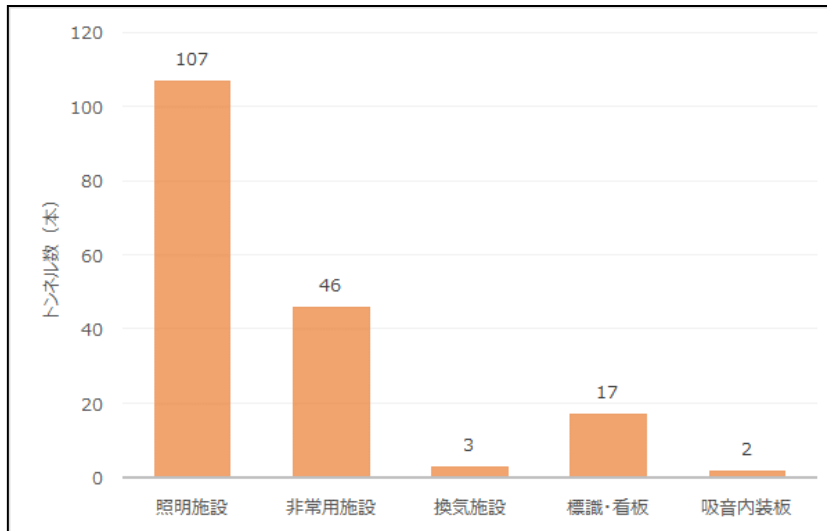
図 2-7 トンネル附属物の状況（令和 5 年 3 月現在）
