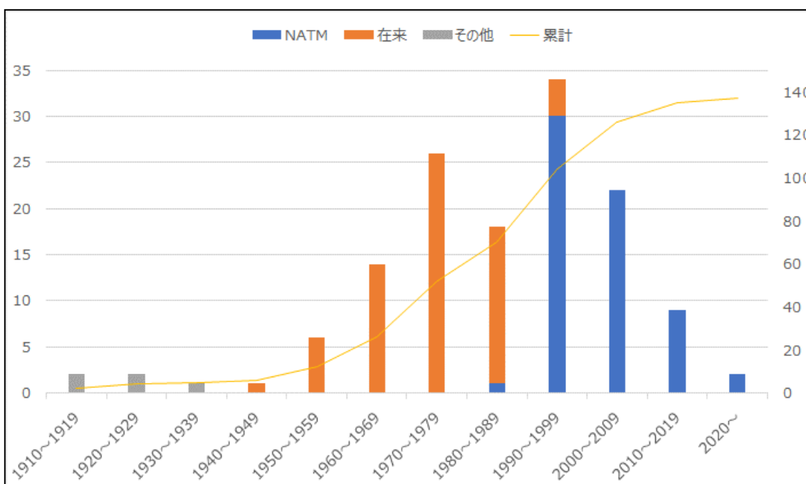
図 2-5 山口県管理トンネルの年度別整備状況（令和 5 年 3 月現在）
