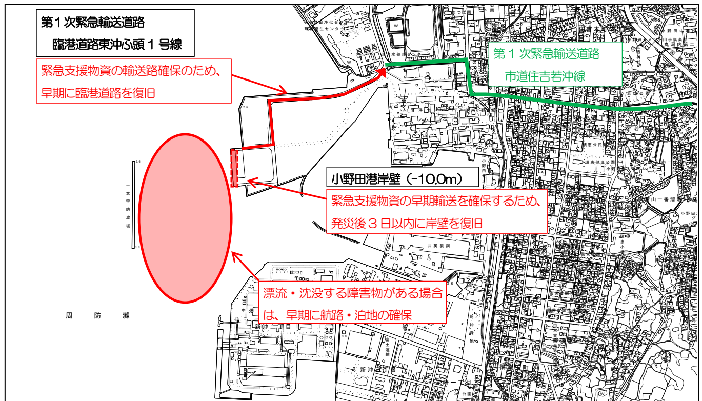
図4-5 小野田港東沖地区の復旧イメージ
