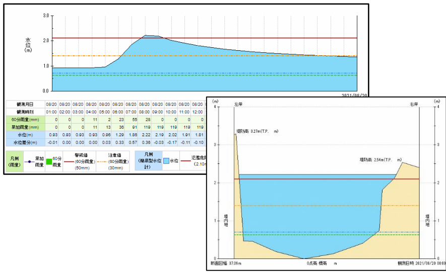
▲簡易型水位計の水位表示の例
