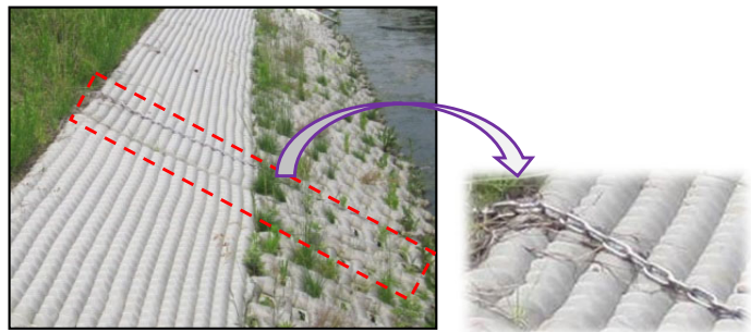
昇降チェーンの設置
