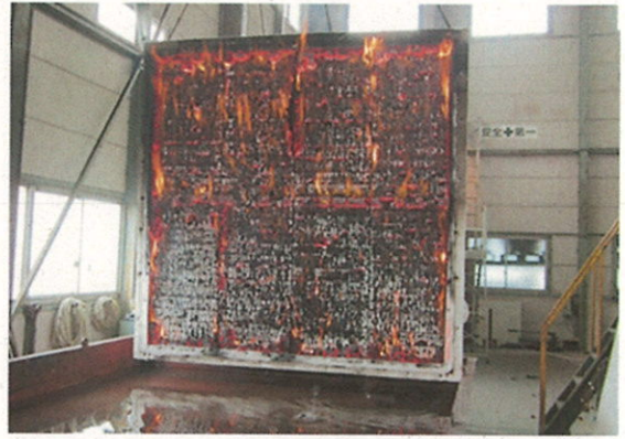
耐火試験
