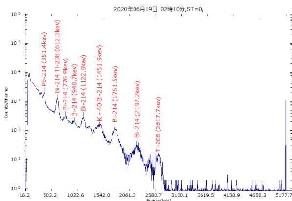
図 3 最高値を観測した時間のスペクトル (2020 年 6 月 19 日 2:10 88.0 nGy/h)
